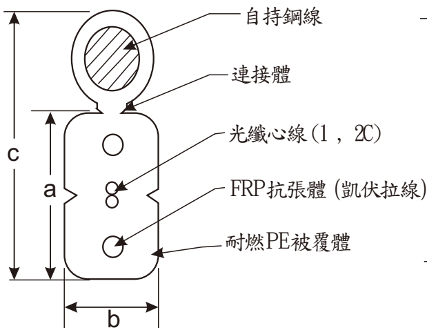
圖1 裸光纖構造圖
