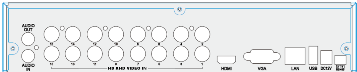
十六路後背板示意圖
