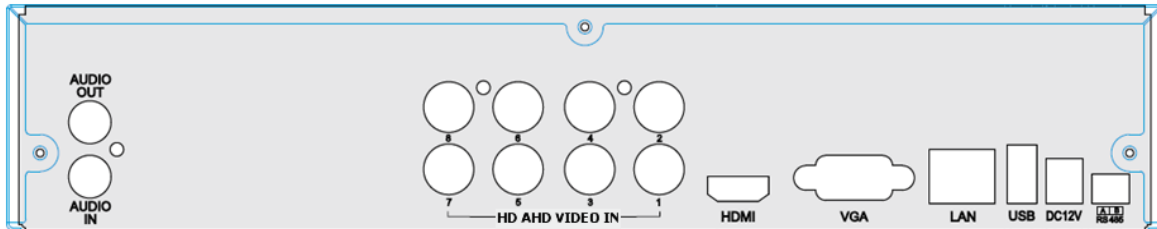
八路後背板示意圖
